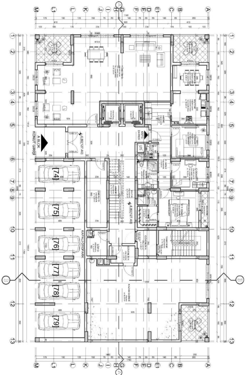
Şekil 5. Mimari Proje 2.Bodrum Kat Planı
