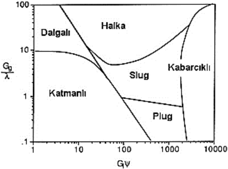
Şekil 12. Yatay boru içinde akış (Baker, 1954; Collier 1996)
