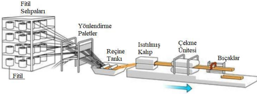
Şekil 4. Pultruziyon yöntemi konfigürasyonu (Marco, 2014)
