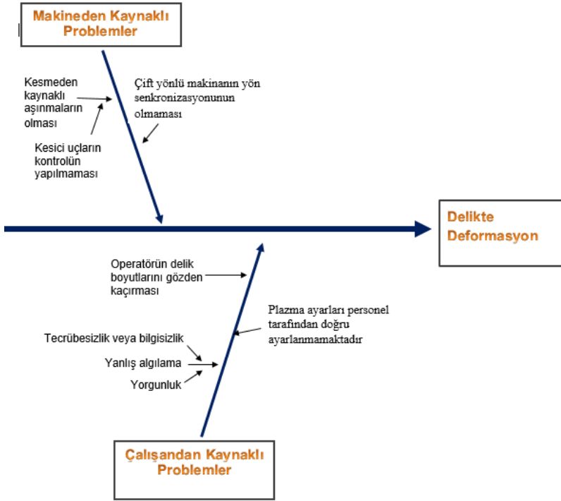
Şekil 6. Delikte Deformasyon Neden Sonuç Diyagramı
