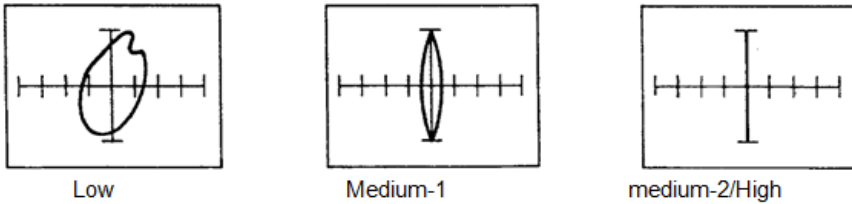
B) 100 \mu F 25V hatalı bir kondansatörün çeşitli aralıklardaki ekran şekilleri
