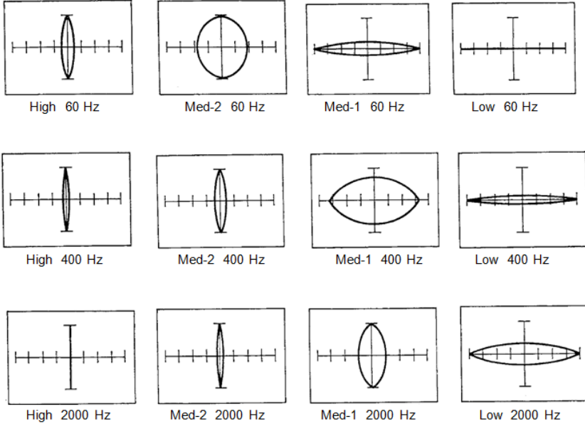
Şekil 21. 0.22 \mu F'lık Bir Kondansatörün Çeşitli Aralık ve Frekanslardaki Test Şekilleri
