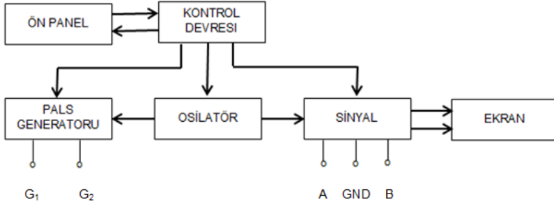
Şekil 14. V-I Test Cihazının Fonksiyonel Blok Diyagramı
