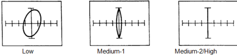
A) 100 \mu F 25V sağlam bir kondansatörün çeşitli aralıklardaki ekran şekilleri
