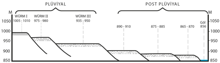
Şekil 8. Pleistosenin plüvyal ve post plüvyal dönemlerde Burdur Gölü havzasında gelişen taraçalar (Erol, 1975'ten)
