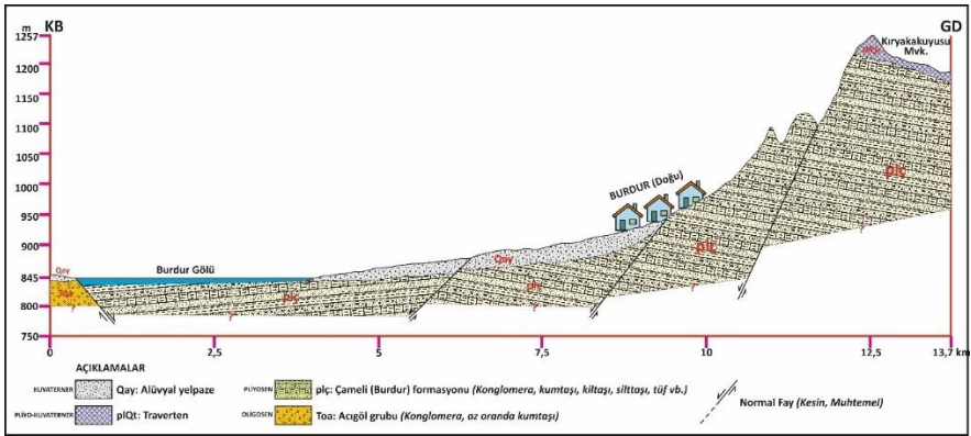
Şekil 2. Burdur şehrinin kurulduğu zemini gösteren jeolojik kesit
