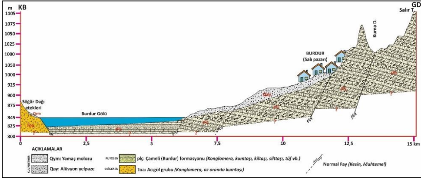
Şekil 7. Söğüt Dağı etekleri - Salır Tepe arasından alınan jeolojik kesit
