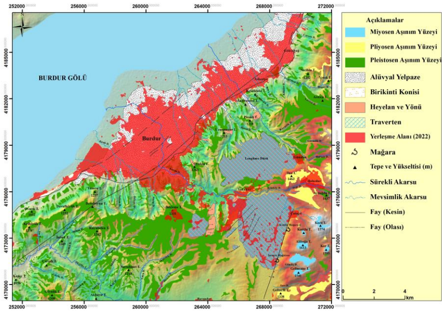
Şekil 5. Burdur ve yakın çevresinin jeomorfoloji haritası
