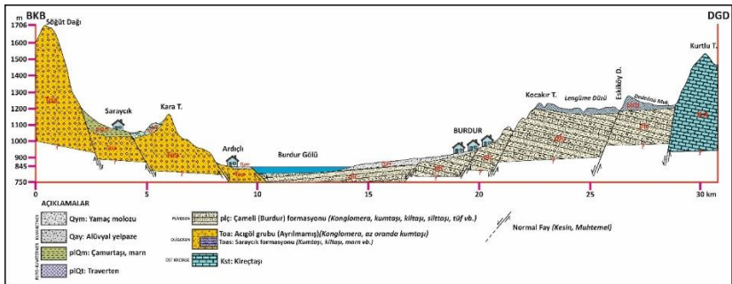
Şekil 6. Söğüt Dağı - Çatağöl güneyindeki Kurtlu Tepe arasından alınan jeolojik kesit
