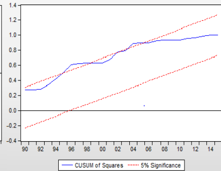
Şekil 2: CusumQ Testi
