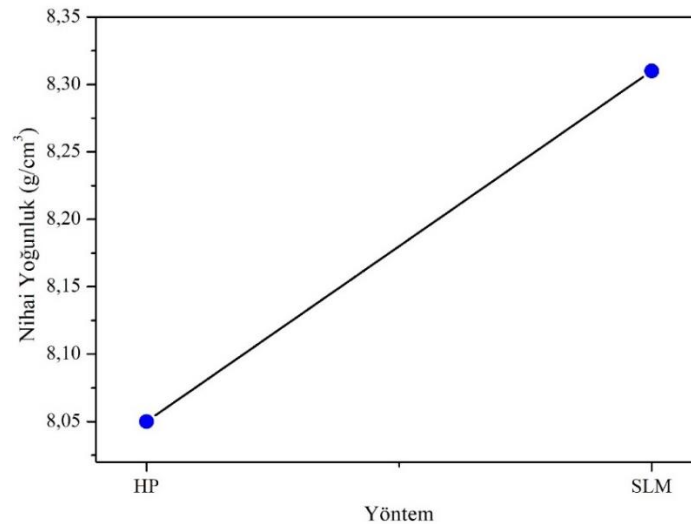
Şekil 4. HP ve SLM ile üretilen numunelerin yoğunluk değerleri
