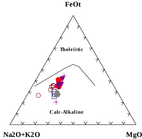
Şekil 58. AFM üçgen diyagramı (Irvine ve Baragar, 1971).
