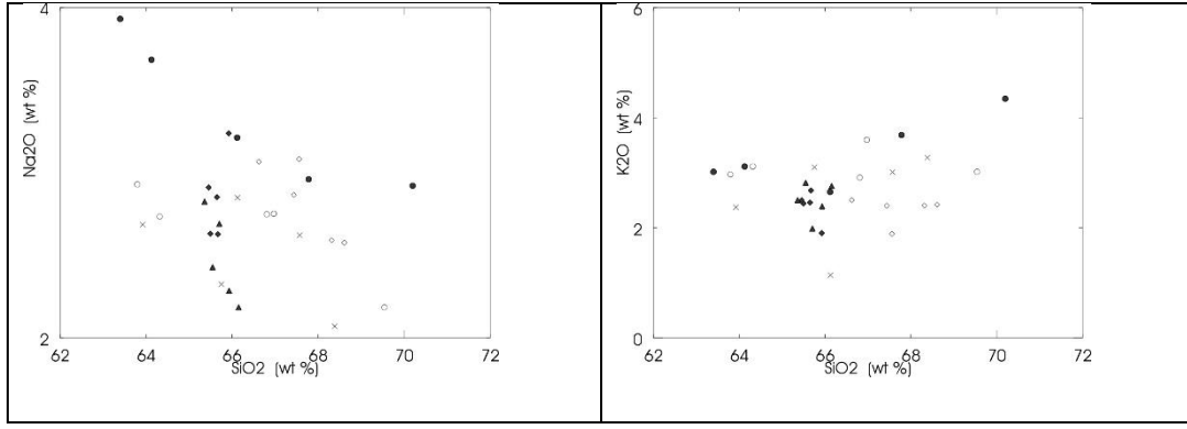
Şekil 59. \text{SiO}_2 ve diğer ana oksit değerlerinin ilişkileri.
