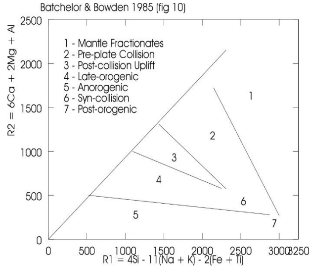
Şekil 34. Granitoidler için çizilmiş örnek bir grafik.
